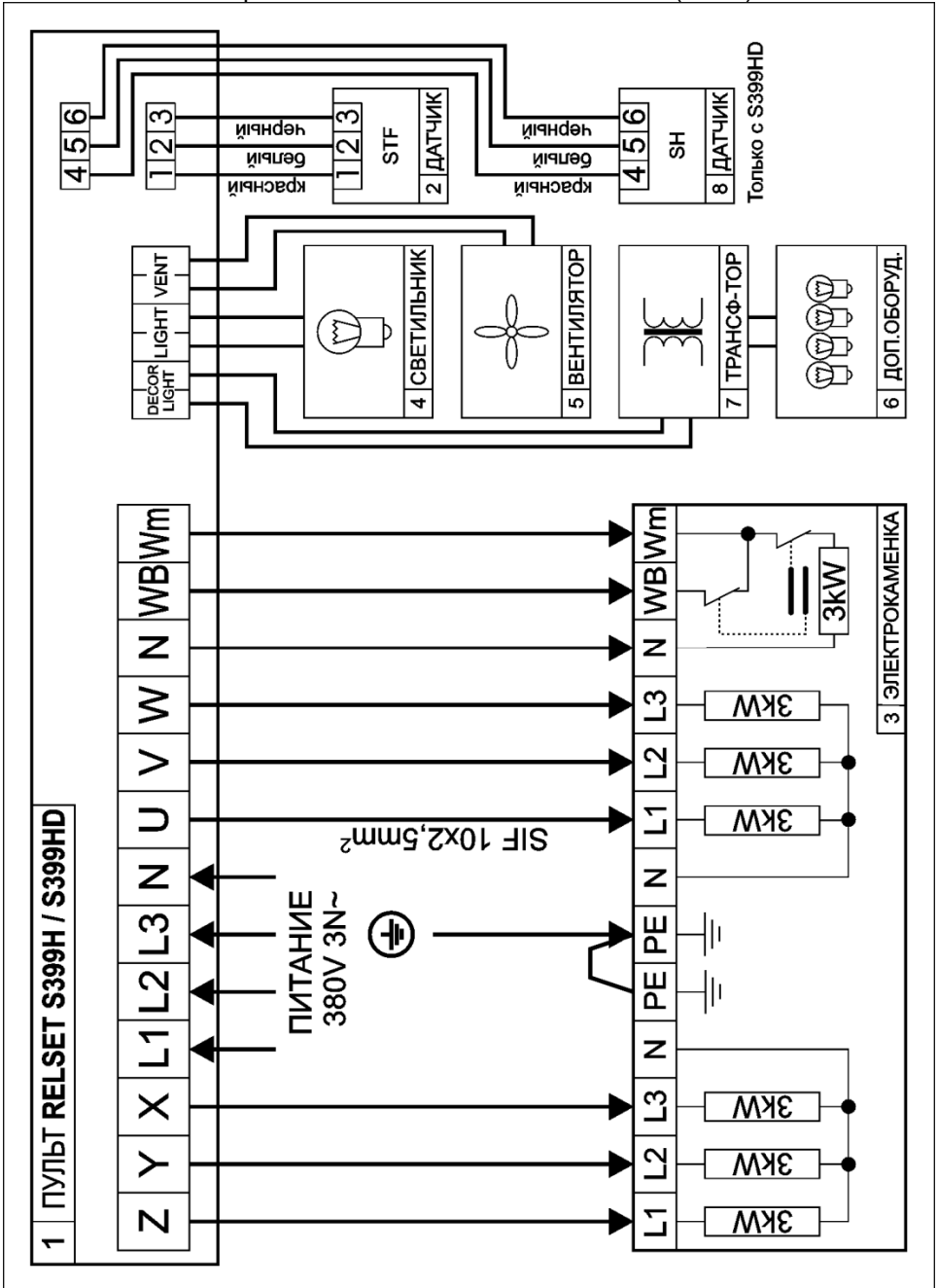
Рис.7 Схема электрическая RELSET S399H / S399HD (380В).
